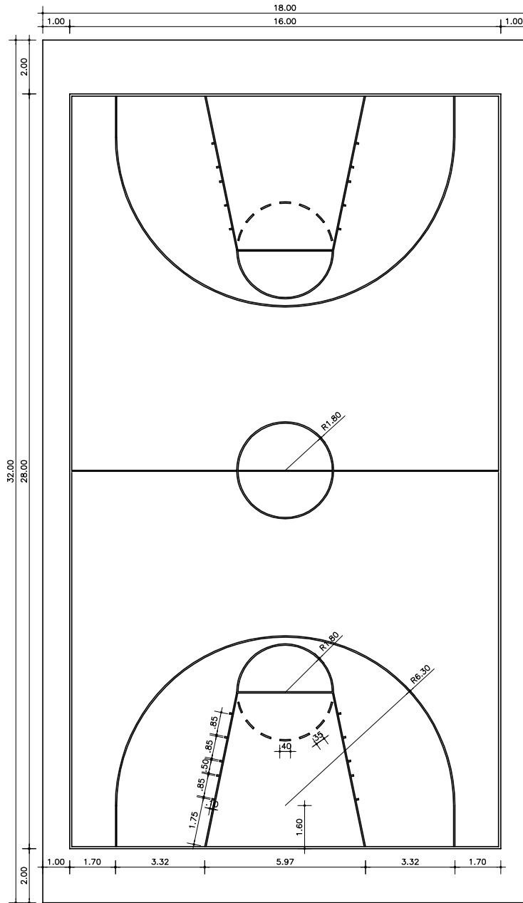
DEMARCAÇÃO DA QUADRA DE BASQUETE
