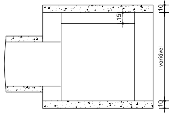
02 CORTE AB ESCALA 1:50
