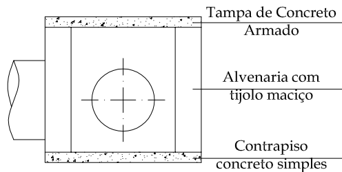
03 CORTE CD ESCALA 1:50
