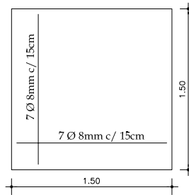
04 TAMPA ESCALA 1:50
