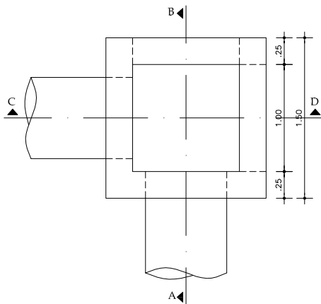
01 PLANTA BAIXA ESCALA 1:50
