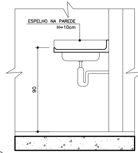
09 Detalhe 1 Esc.: 1:25
