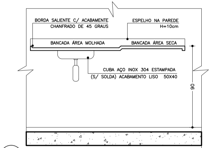
10 Detalhe 2 Esc.: 1:25
