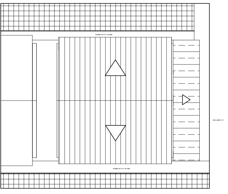
Planta de Cobertura, locação
