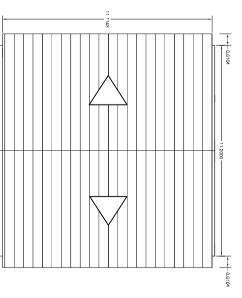
Planta de Cobertura
