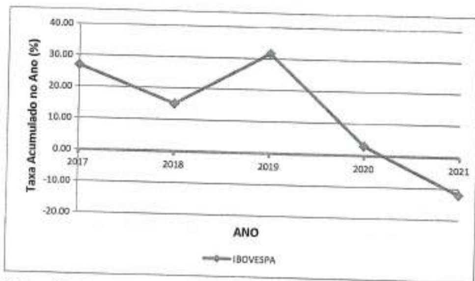
Gráfico 10 – Rentabilidade IBOVESPA (%) – 2017/2021
