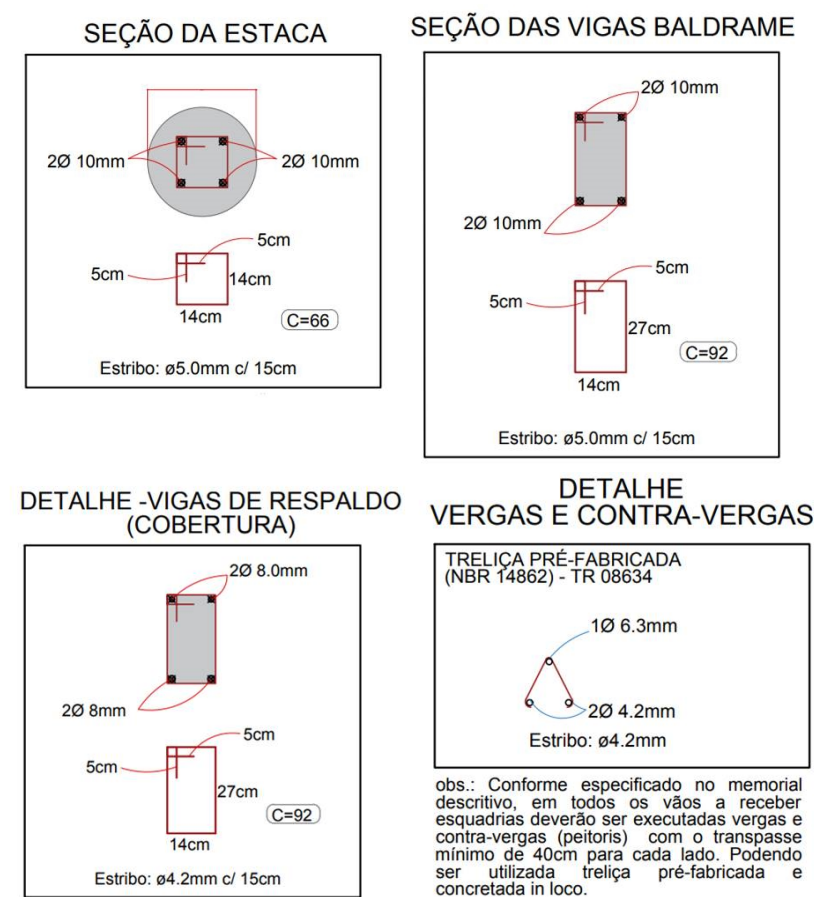
DETALHE DE FERRAGENS esc: indicada
