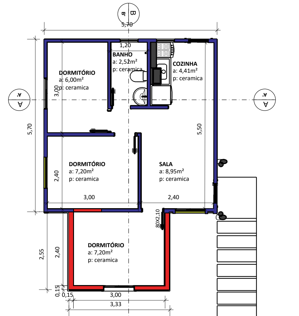
PLANTA BAIXA TÉCNICA - esc:1/75
