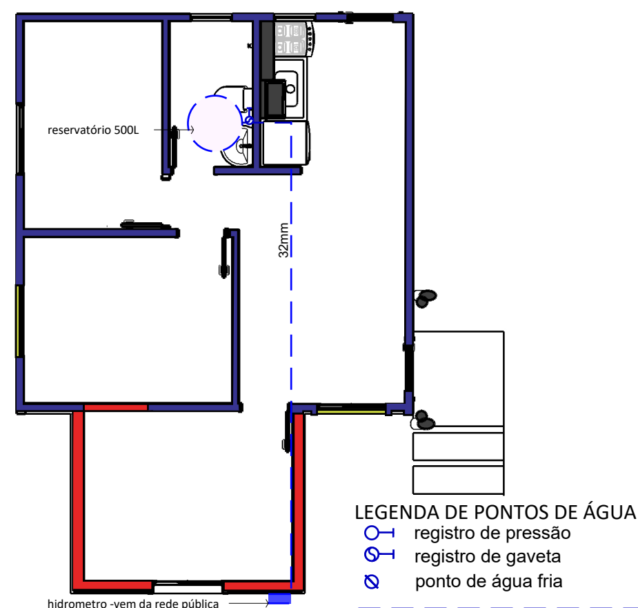
HIDROSSANITÁRIO - esc:1/75
