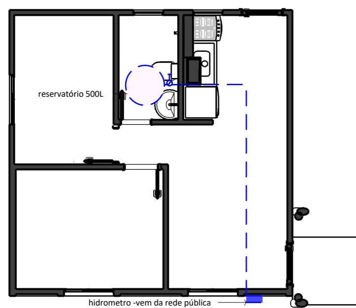
PLANTA BAIXA - esc:1/75
