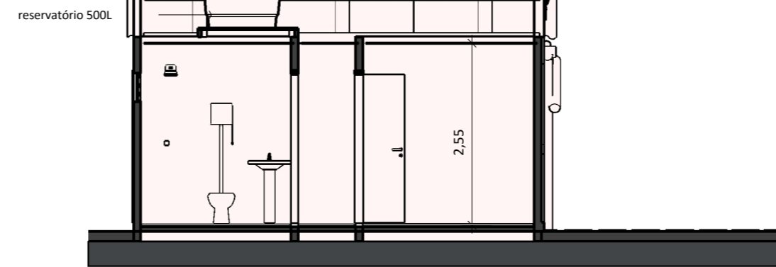
CORTE B, B' - esc:1/75
