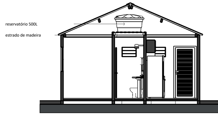
CORTE A, A' - esc:1/75
