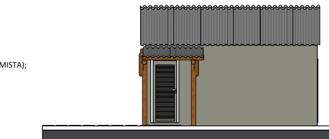
FACHADA LATERAL DIREITA - esc:1/75
