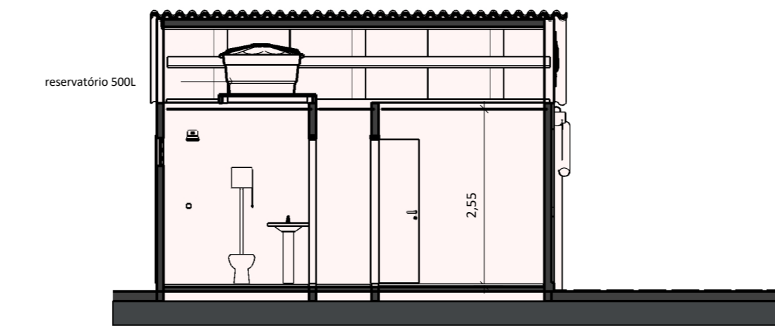
CORTE B, B' - esc:1/75
