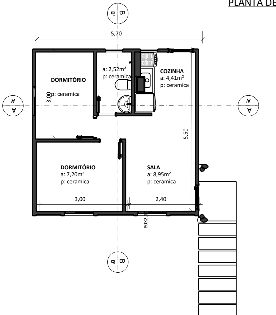
PLANTA BAIXA - esc:1/75
